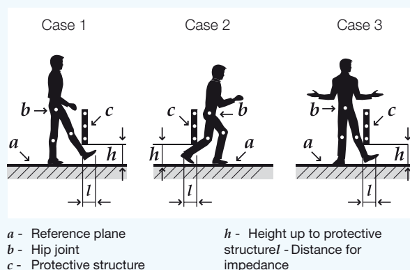
□ FIGURE A.1 (EN ISO 13857)
